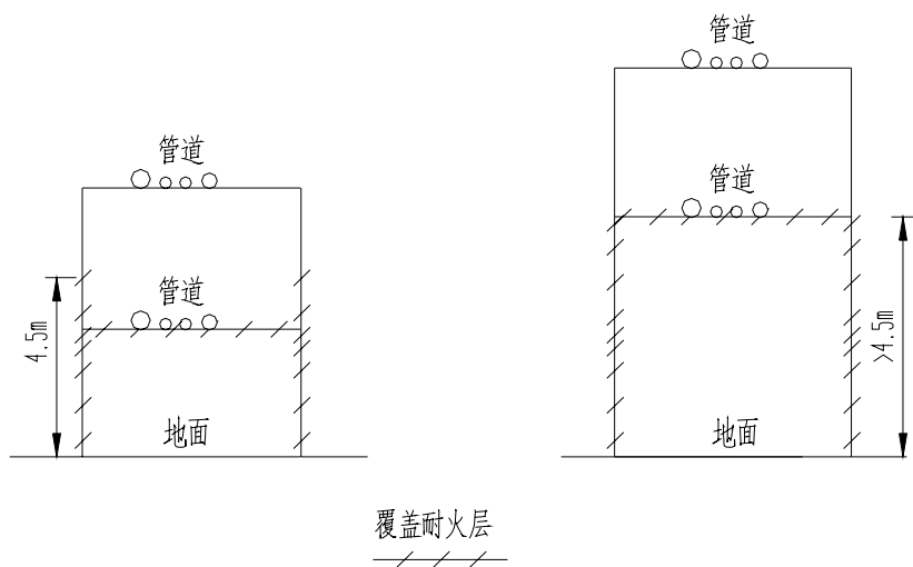
图 6 钢管架 I
